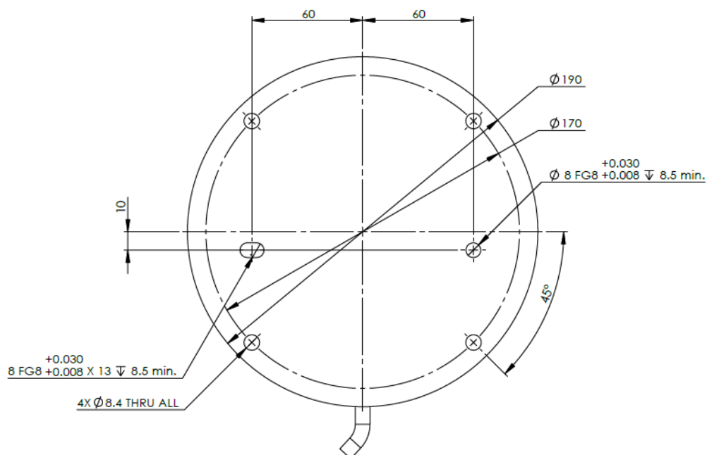
1.1: Vedea de jos bazei robotului
