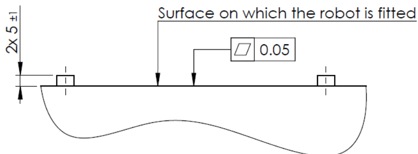
1.2: Placă de montare pentru baza robotului
